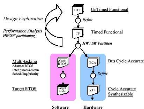
Niveaux d'abstraction SystemC (source : OSCI)
